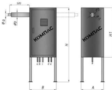
Рисунок 1 – Габаритные размеры котлов
